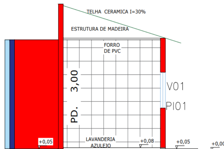
CORTE A A' ESC. 1:100
